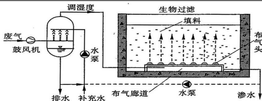
图 6.2.1-3 生物滤池示意图
