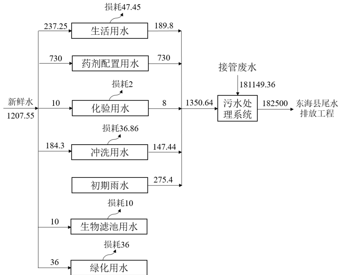
图 3.1.4-1 本项目水平衡图
