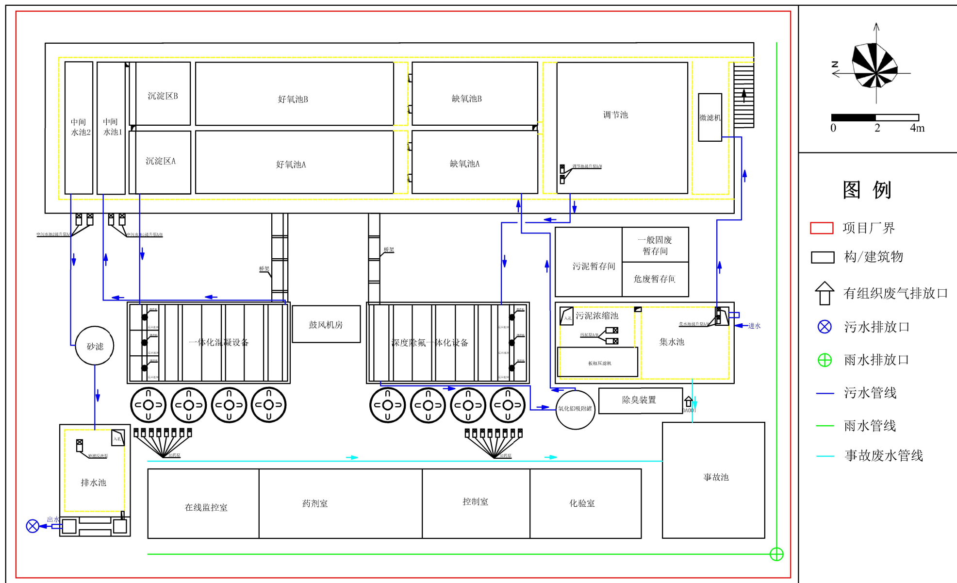
图3.1.5-1 厂区平面布置图
