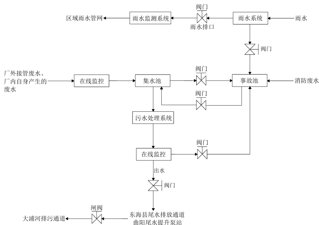
图 6.2.7-1 防止事故废水进入外环境的控制、封堵系统图
