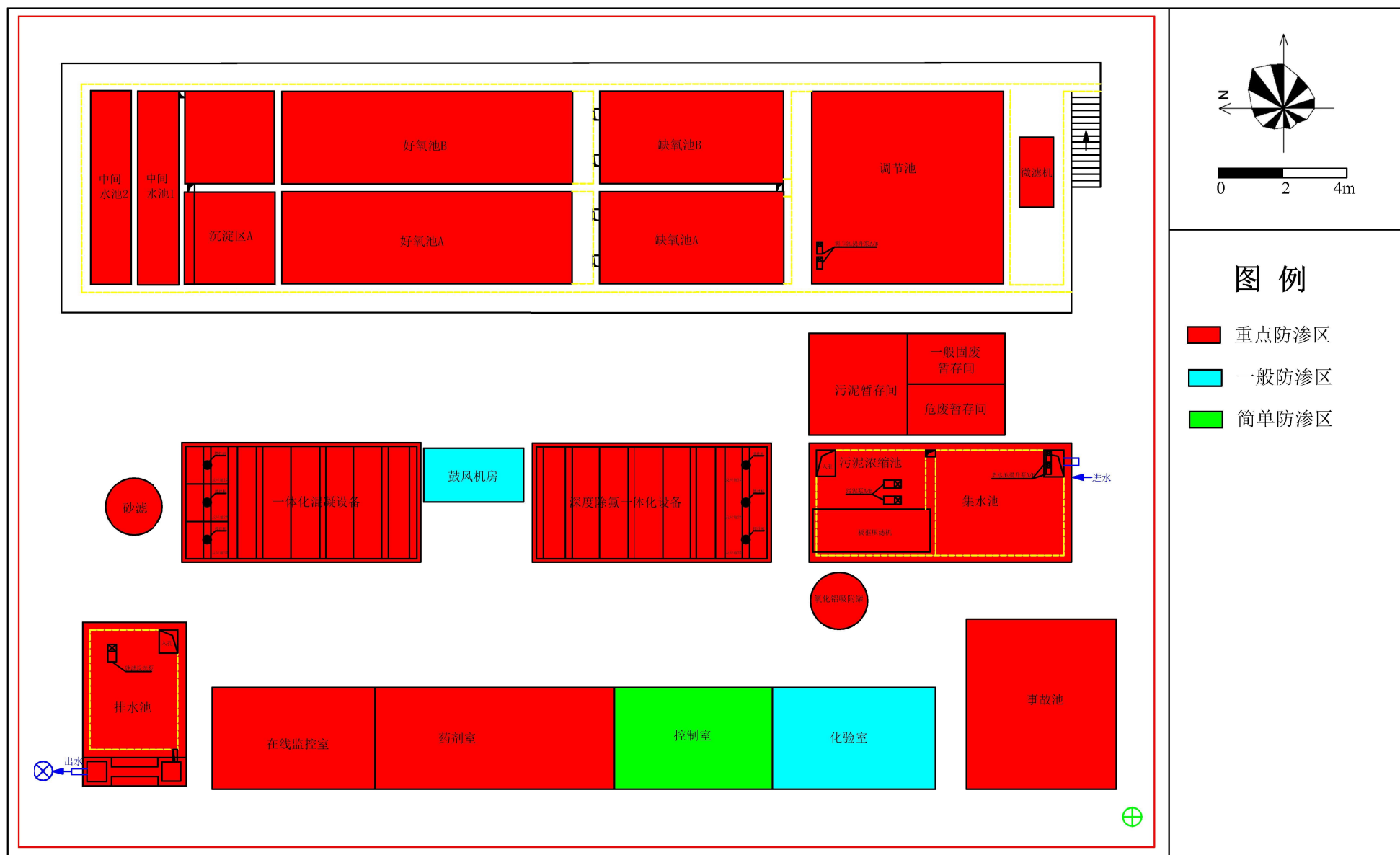
图6.2.3-1 厂区分区防渗图
