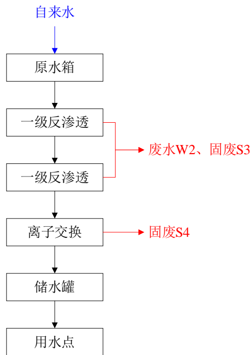
图2-3 纯水制备生产工艺流程及产污环节图
