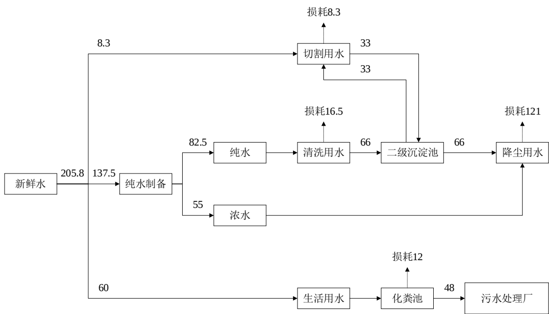
图2-1 本项目水平衡图（单位：m³/a）
