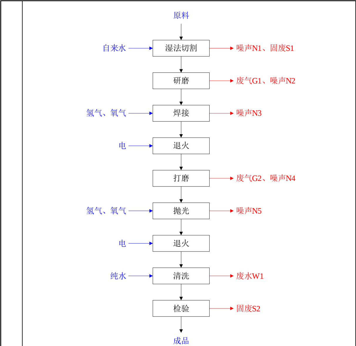
图2-2 半导体用石英玻璃器件生产工艺流程及产污环节图
