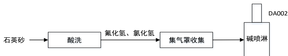
图 4-2 废气处理流程图
