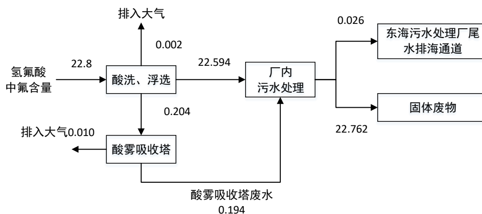
图 2-4 本项目氟平衡图 (t/a)
