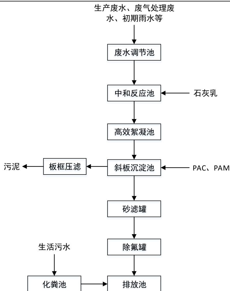
图 4-1 生产废水处理工艺流程图
