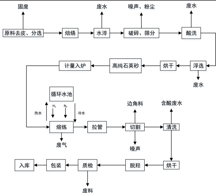
图2-6 石英玻璃管生产工艺及产污环节图
