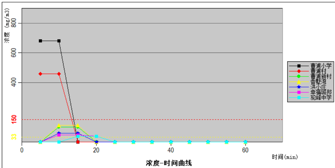
图 3.3-3 最不利气象条件下敏感点氯化氢浓度随时间变化情况图
